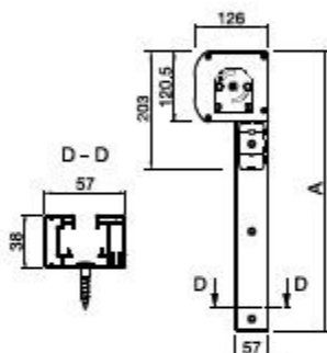
Leibungsmontage mit Befestigungsbohrer (breite Führung) Montaggio in luce con fori di fissaggio (guida larga) A = Total Höhe / A = Altezza totale
