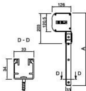
Leibungsmontage mit Befestigungsbohrer (schmale Führung) Montaggio in luce con fori di fissaggio (guida sottile) A = Total Höhe / A = Altezza totale
