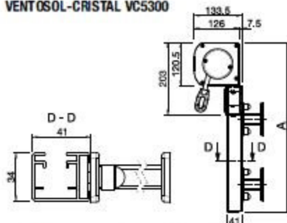
Aufgesetzte Wandmontage mit Befestigungshalter Montaggio a parete con piastra di fissaggio A = Total Höhe / A = Altezza totale
