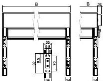
Montageplan mit Befestigungshalter Schema di montaggio con piastra di fissaggio B = Total Höhe / B = Altezza totale
